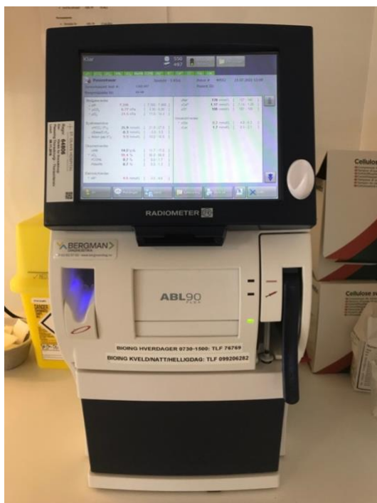
Figur 9: "Bedside" blodgassanalyseapparat Radiometer ABL 90 på Thorax Intensiv
